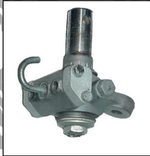
No. DE PARTE 636 REPUESTO PARA VALVULA TIPO SCANIA 1726573
