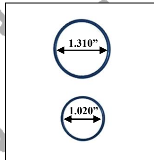
No. DE PARTE 557 REPUESTO PARA INYECTOR TIPO SCANIA
