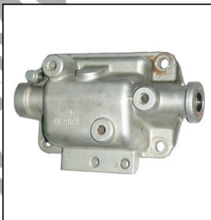
No. DE PARTE 603 REPUESTO PARA TAPA DE TORRE DE CAMBIOS TIPO 3316416
